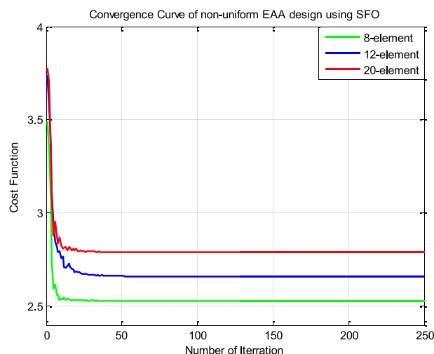
Figure 20. Convergence plots of EAAs.
