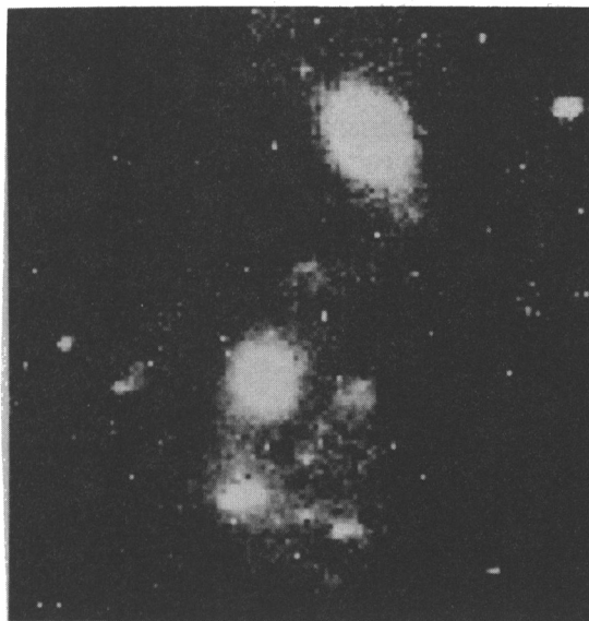
Fig.3c Arp143 (K-Band)
