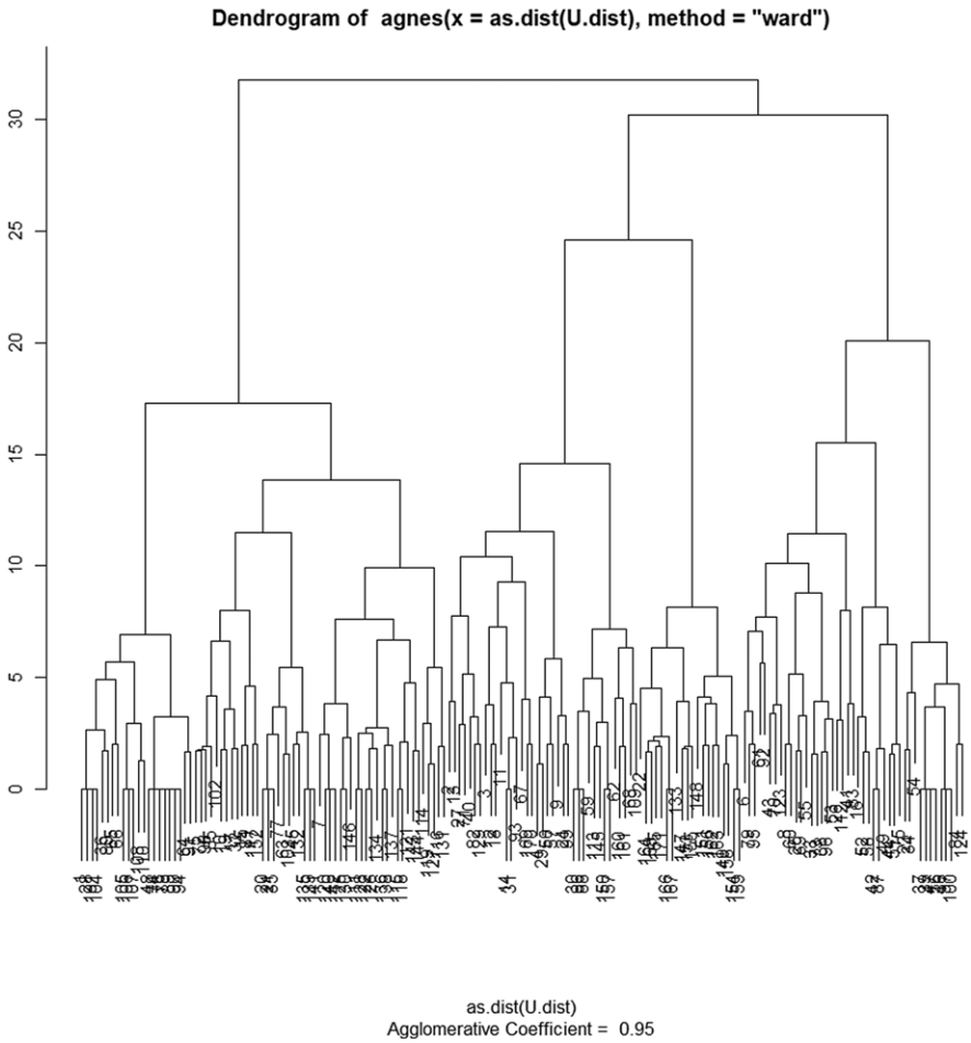
A1. Dendrogram.
