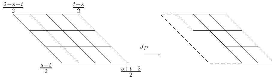
FIGURE 1. Représentation graphique de [\overrightarrow{3}]_{[\overleftarrow{4}]_\pi} ainsi qu'un des constituants de son image par J_{P_{6g,19g}^{op}} .
