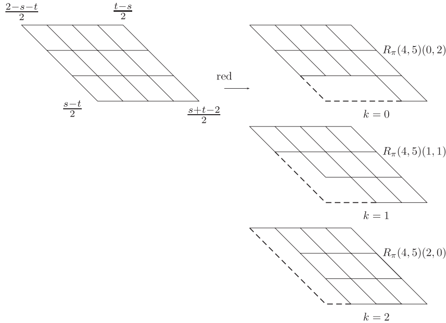
FIGURE 2. Illustration graphique du corollaire 1.5.6 dans le cas r = 3 avec (s, t) = (4, 5) .
