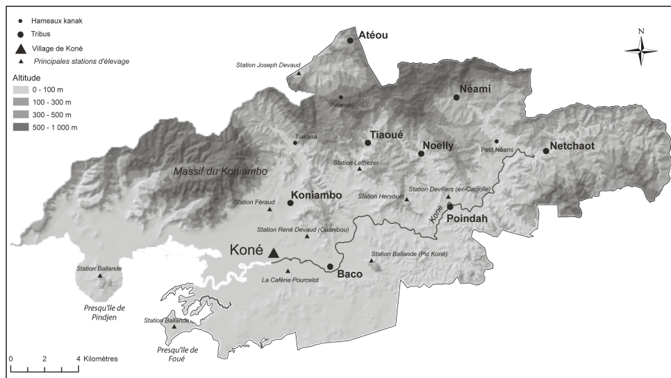
Figure 4 – Carte de la commune de Koné dans l'entre-deux-guerres
