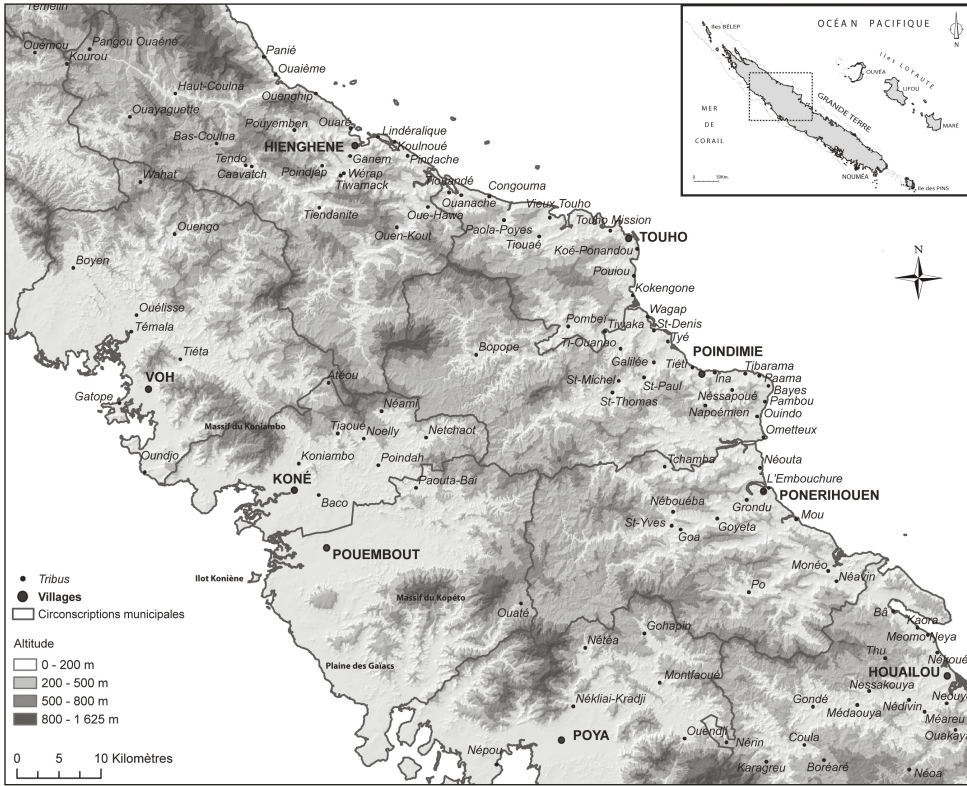
Figure 2 – Carte du centre-nord de la Grande Terre de Nouvelle-Calédonie
