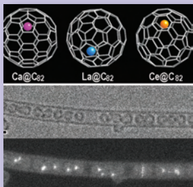
Ca metallofullerene peapod K. Suenega, AIST
